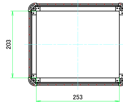
C-C ( 1 : 5.5 )
