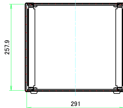
A-A ( 1 : 5.5 )
